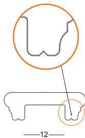
Gocciolatoio
