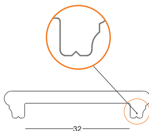
Gocciolatoio
