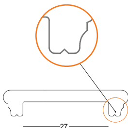
Gocciolatoio
