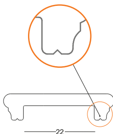
Gocciolatoio
